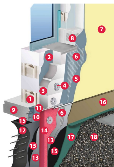
Рис. 5. Система фасадного утепления стен ЛСР ТЕРМО
