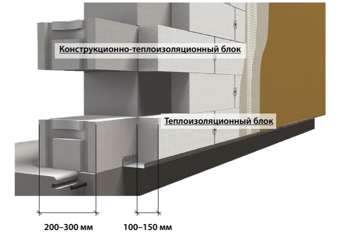
Рис. 4. Энергоэффективные двухслойные стены из газобетона с внешним утеплением ЛСР ТЕРМО
