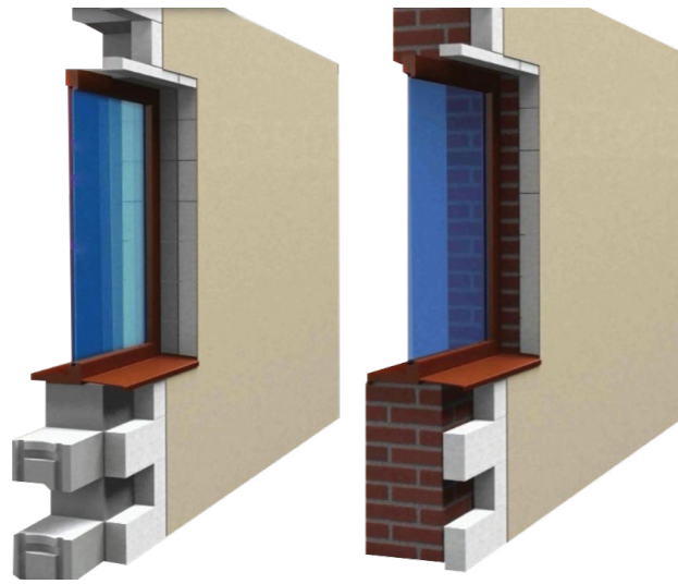
Рис. 2. Система фасадного утепления ЛСР ТЕРМО
