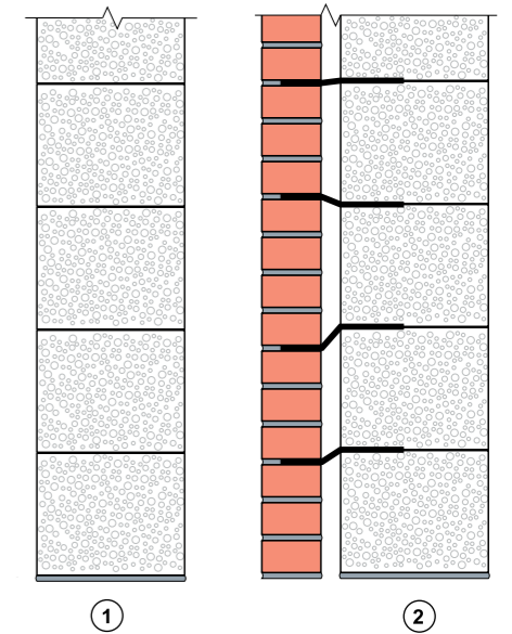
Рис. 4.3. Схемы стен из блоков ЛСР: 1 — однослойная; 2 — двухслойная
