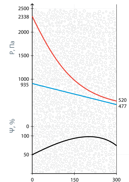
Давление реального и насыщенного водяного пара в толще стены
