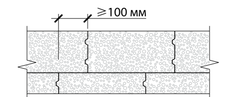
Рис. 4.4. Перевязка кладки
