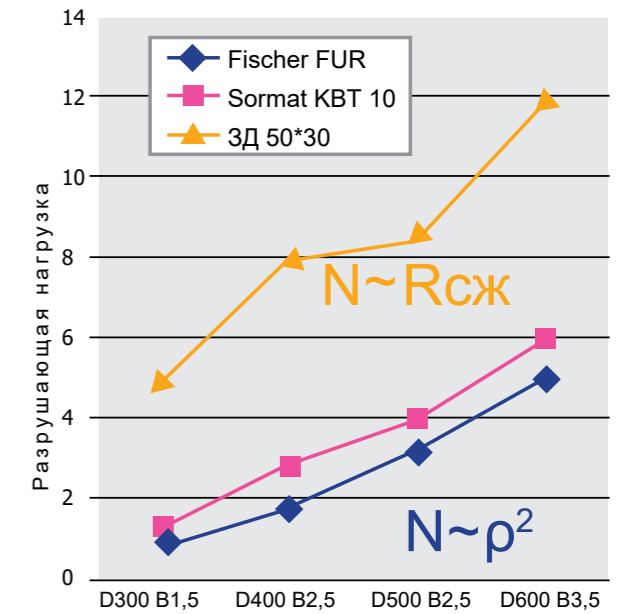
Зависимость несущей способности крепежа от формы дюбеля и плотности газобетона
