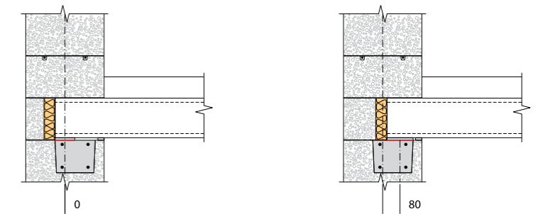
В – опирание на центрирующие прокладки
