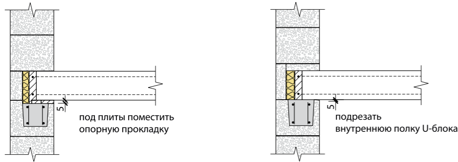
Рис. 4.12. Варианты перекрытий по стенам из блоков ЛСП
