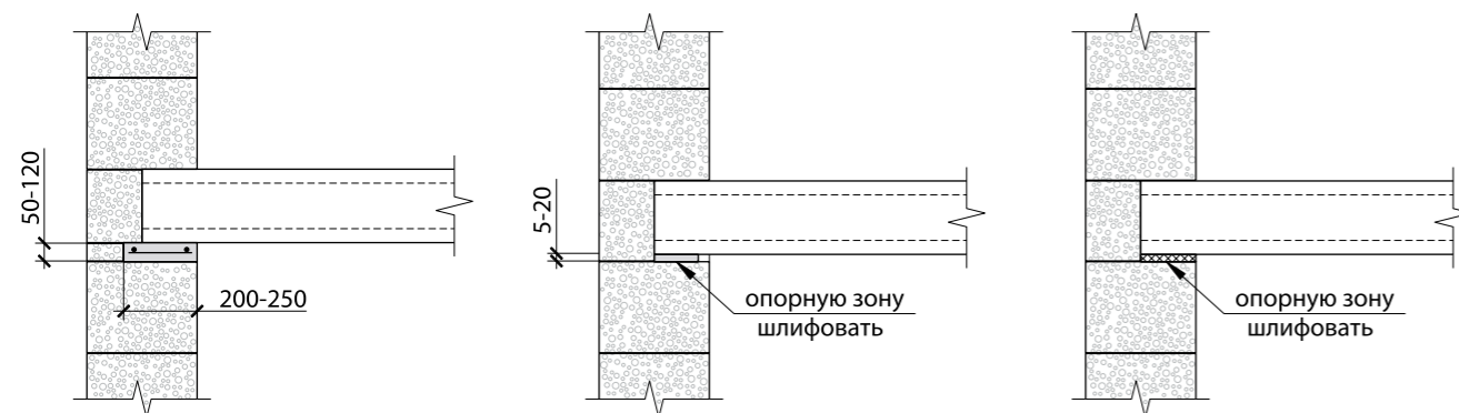
Рис. 4.13. Варианты перекрытий по стенам из блоков ЛСП
