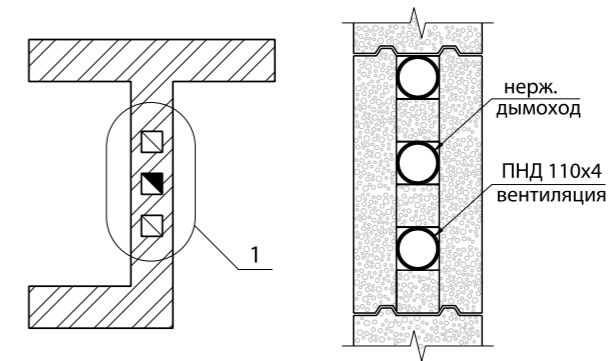
Рис. 4.6. Пример устройства вентиляционных стояков и дымоходов в кладке из блоков ЛСР
