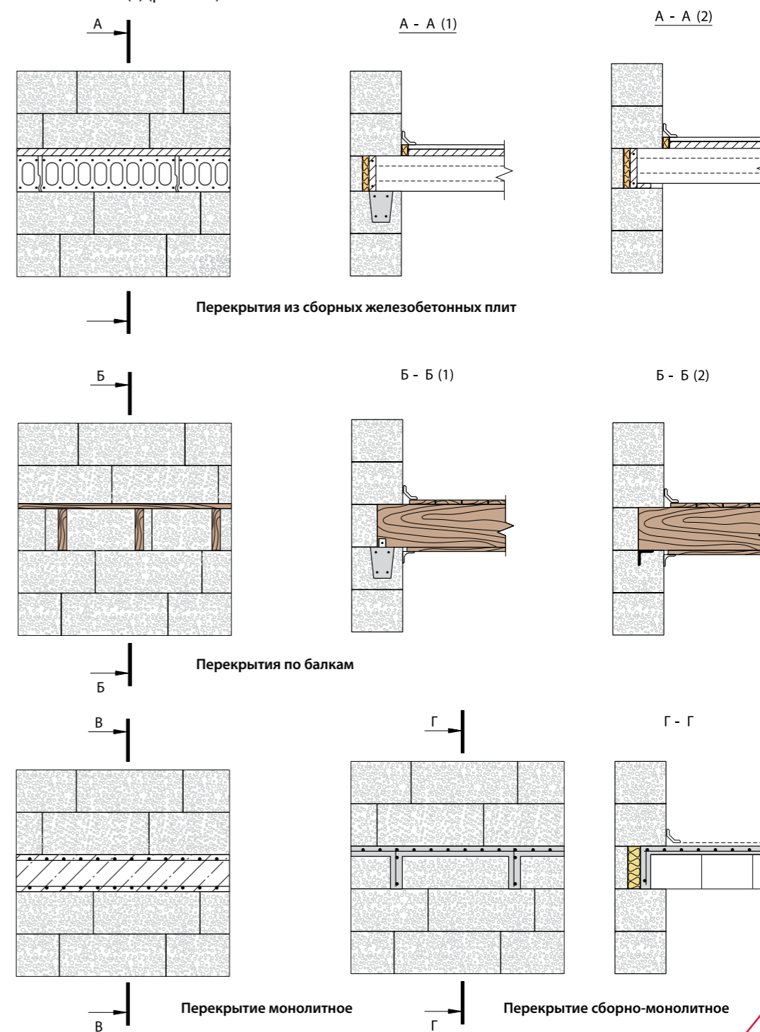
Рис. 4.11. Варианты перекрытий по стенам из блоков
