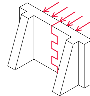
Рис. 3.3. Растяжение кладки при изгибе по перевязанному сечению
